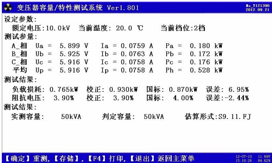
图 7、容量测试结果
