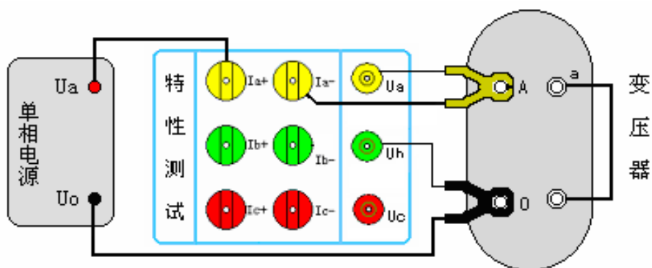
图 26、单相变压器短路损耗测量
