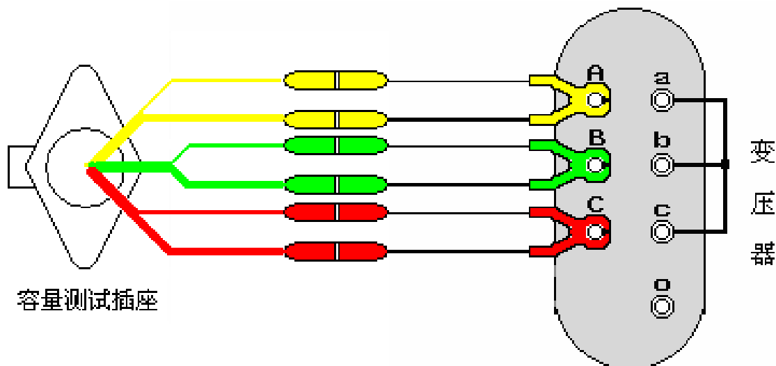
图 24、容量测试接线示意图
